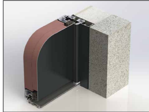
Pose en applique
