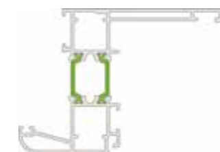
Dormant RENOVATION avec aile de 60 mm Mars 2018
